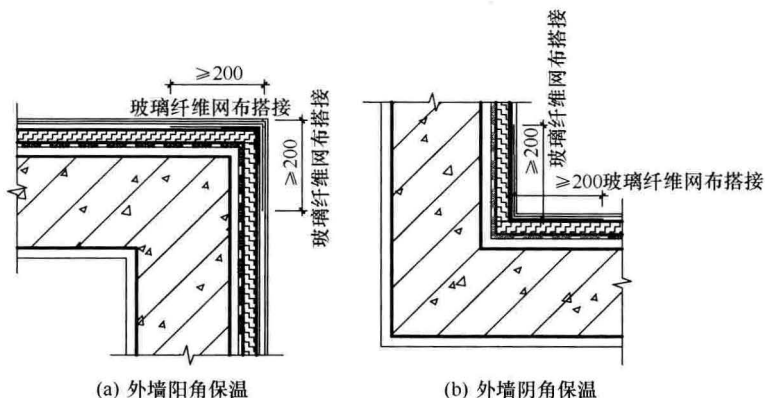
图 6.2.5 外墙阳角、阴角保温
