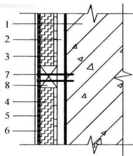
图 6.2.9 龙骨面板外墙 内保温系统
