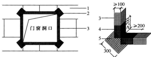
图 7.2.8 门窗洞口玻璃纤维网布加强示意图
