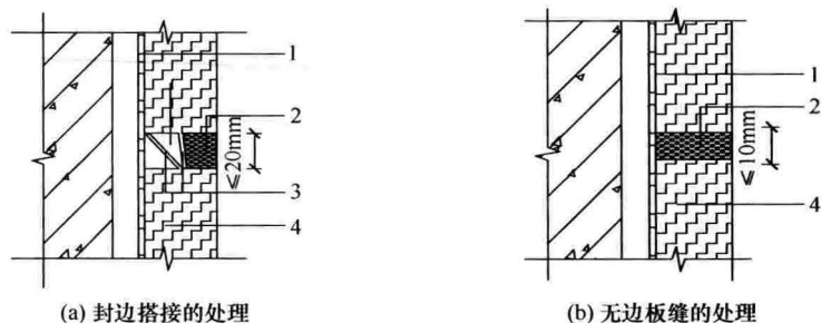
图 7.2.5 真空绝热板板缝施工示意图
