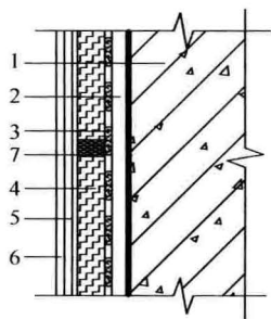
图 6.2.8 薄抹灰外墙 内保温系统
