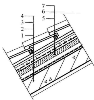
图 6.2.16-4 倒置式坡屋面 保温系统
