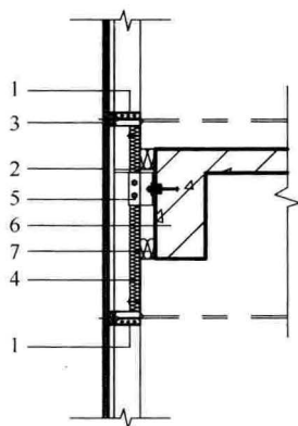
图 6.2.34-2 复合玻璃幕墙板系统竖剖构造
