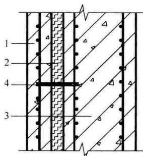
图 6.2.23 复合预制墙板构造
