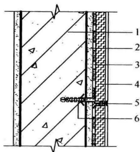
图 6.2.11 保温装饰板外墙 外保温系统构造
