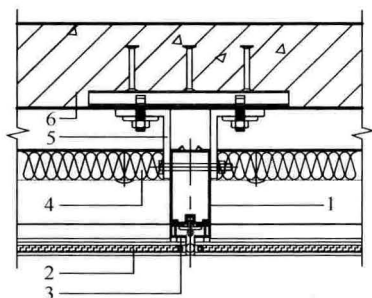
图 6.2.34-1 复合玻璃幕墙板系统横剖构造
