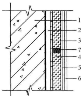
图 6.2.1 薄抹灰外墙外保温系统构造
