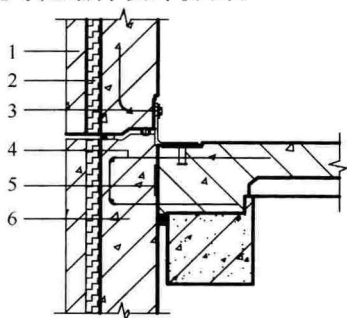
图 6.2.29 复合预制墙板预埋件布置图
