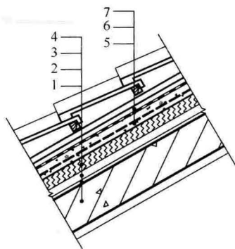
图 6.2.16-3 正置式坡屋面 保温系统
